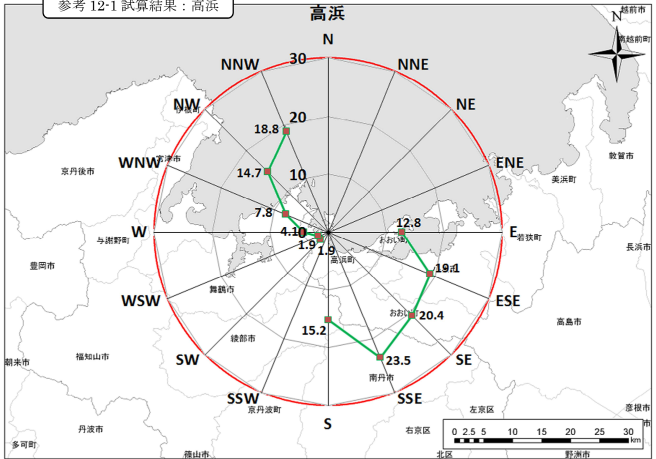
参考 12-1 試算結果：高浜
