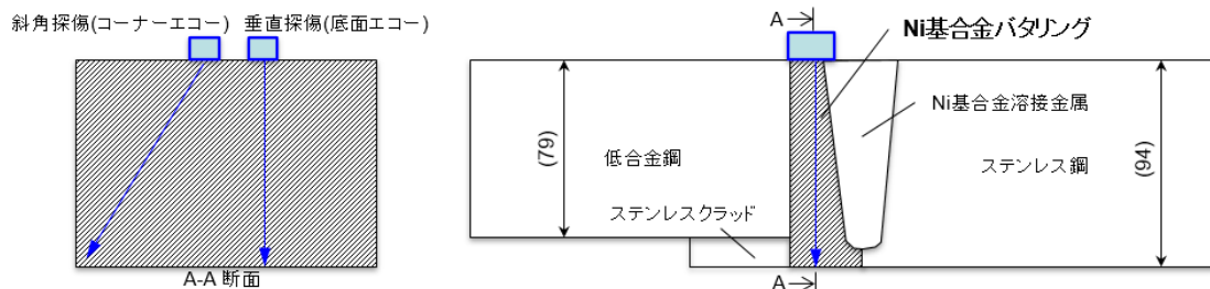
図 1 厚板継手溶接試験体
