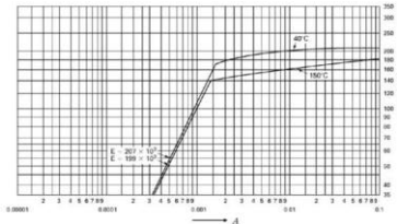
Part 3 第3章 図5 炭素鋼及び合金鋼 (それぞれ常温最小降伏点が410MPa以上のもの)
