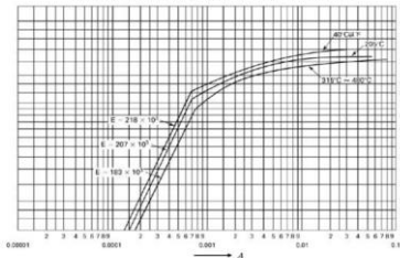
Part 3 第3章 図10 高ニッケル合金 (GNCF690HYSU)
