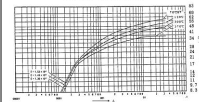
Part 3 第3章 図15 白銅 (C7150)
