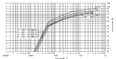
Part 3 第3章 図18 高ニッケル合金(NW4400)
