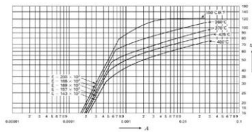
Part 3 第3章 図3 炭素鋼(常温最小降伏点が210MPa以上410MPa未満のもの)及び ステンレス鋼(SUS410及びSUS410T1TB)
