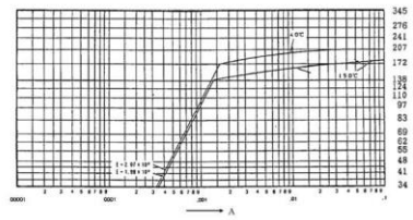
Part 3 第3章 図5 炭素鋼および合金鋼 (それぞれ常温最小降伏点が410MPa以上のもの)
