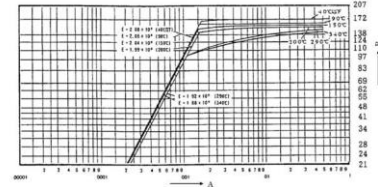
Part 3 第3章 図6 低合金鋼 (SQV1A, SQV2A, SQV2B, SFVQ1A, SFVQ1B及びSFVQ2A)
