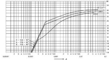
Part 3 第3章 図16 白銅 (C7060)
