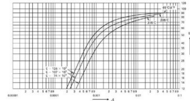
Part 3 第3章 図17 アルミニウム青銅 (C6161及びC6280)
