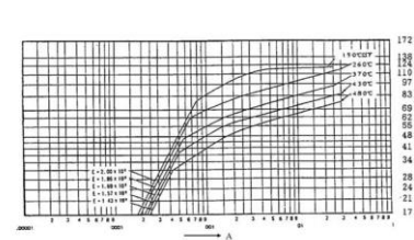
Part 3 第3章 図3 炭素鋼(常温最小降伏点が210MPa以上410MPa未満のもの)及び ステンレス鋼(SUS410及びSUS410T1TB)
