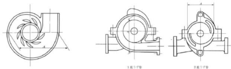
図 PMO-3320-3 うず巻ポンプであって、ケーシングが軸垂直割りで案内羽根を有するもの
