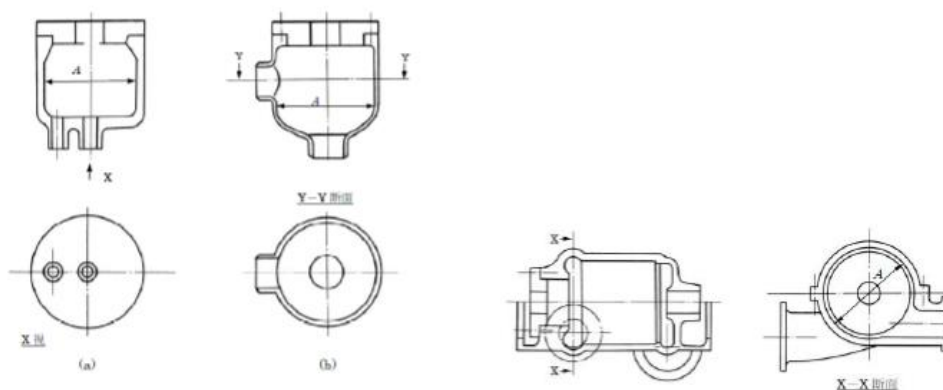
図 PMO-3320-5 ターボポンプであって、ケーシングが軸垂直割りで軸対称であるもの
