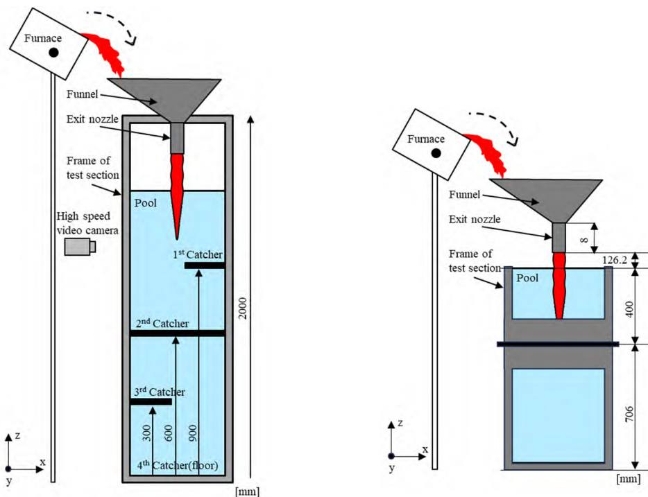
(a)DEFOR-A 実験装置
