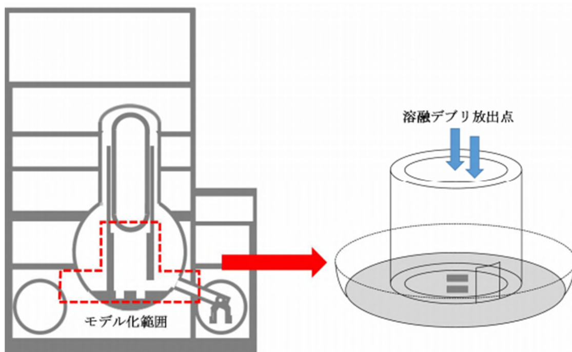
図 4-4 代表的な BWR 解析体系
