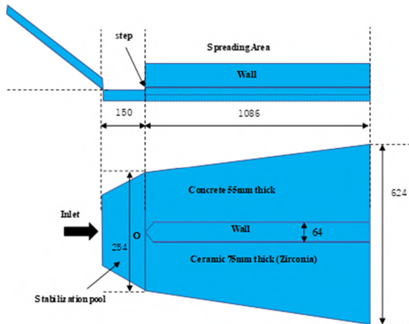
図 4-3 VULCANO-VEU7 解析体系
