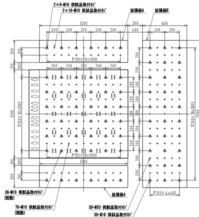
図 2 振動台テーブルの図面
