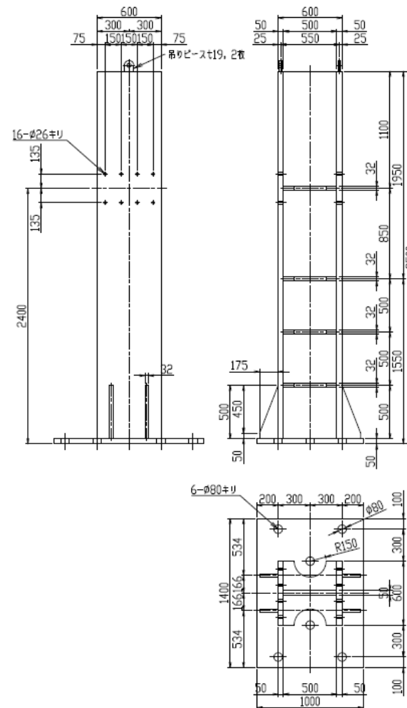
図 5 反力支柱
