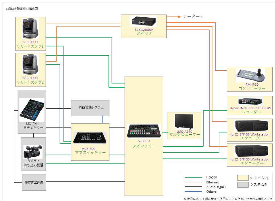
(13F A 会議室機材構成図)
