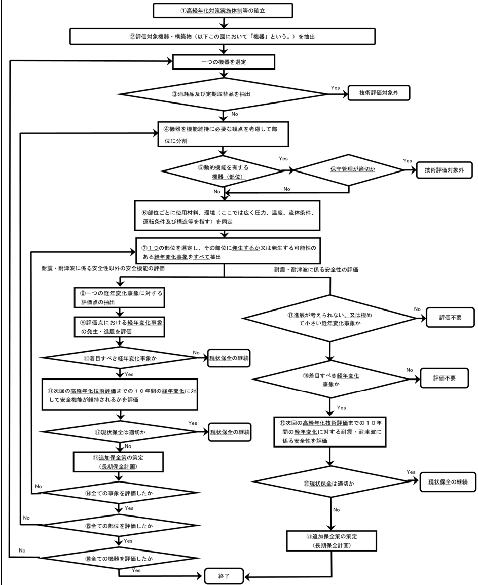
別図 高経年化技術評価の基本的な流れ
