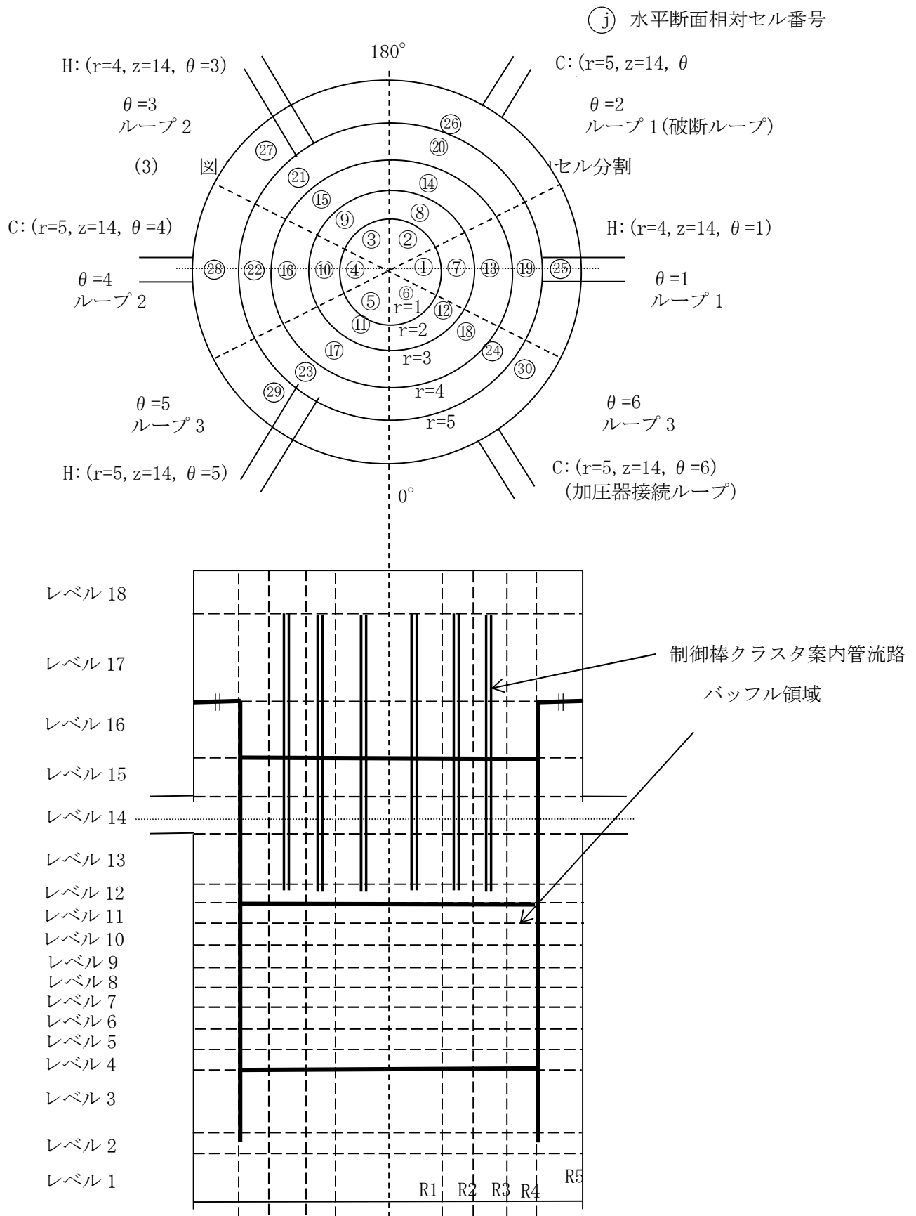
図2 PWR 3 ループプラントの原子炉容器内の炉心領域を除くセル分割
