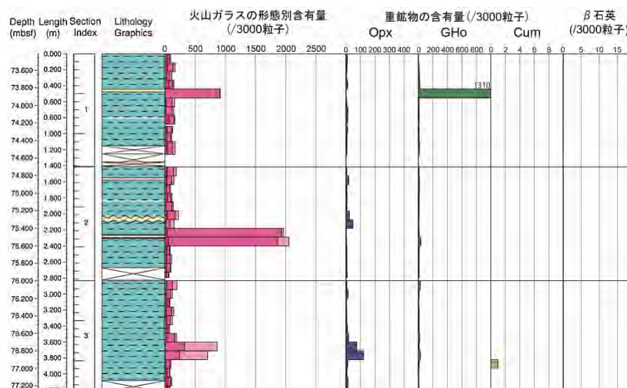
図 4.2.1 層準別ヒストグラムの参考図
