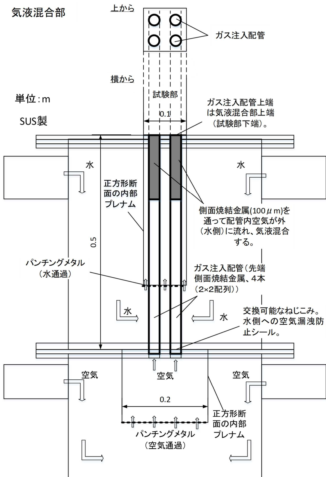
図4 気液混合部参考模式図
