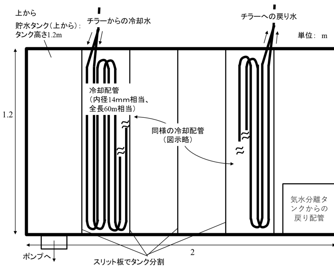
図3 貯水タンクと冷却システムの参考模式図 (上面図)
