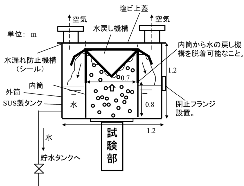
図2 気水分離タンクと噴き出し水の戻し機構の参考模式図
