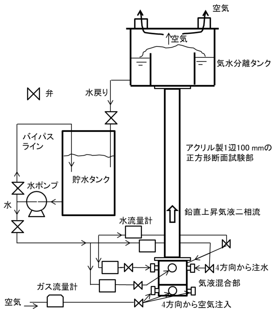
図1 既設気液二相流のガス移行実験装置の模式図
