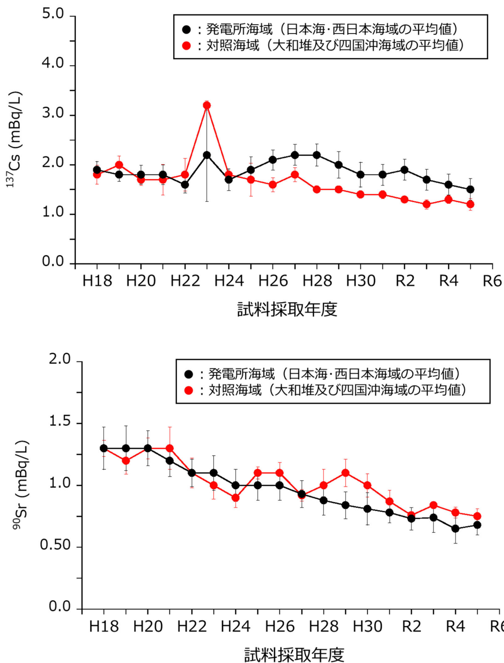
図 I -2-2-1-7 発電所海域（日本海・西日本海域）及び対照海域（大和堆及び四国沖海域）の表層で採取した海水試料に含まれる ^{137}\text{Cs} と ^{90}\text{Sr} 濃度の平均値の経年変化（誤差棒は各年度の標準偏差を示す。）
