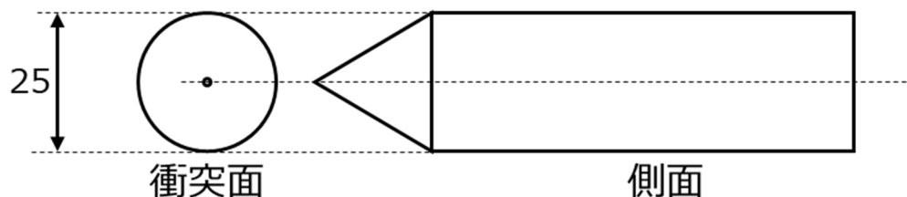
図2 衝突物イメージ（単位：mm）
