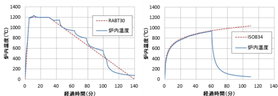
図 2 加熱装置の加熱曲線の一例
