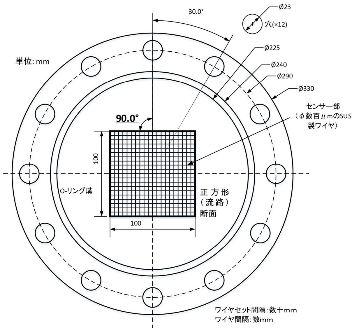
図1 ワイヤメッシュセンサーの模式図（ワイヤは実際の一部のみ模式的に描写）
