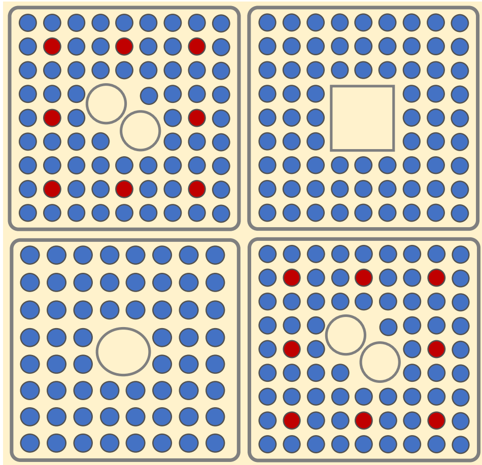
図1 8×8及び9×9燃料集合体装荷炉心（混在炉心事例）
