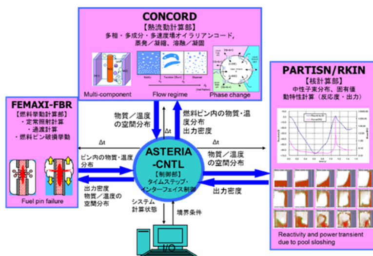
図 1 ASTERIA-SFR のコード構造
