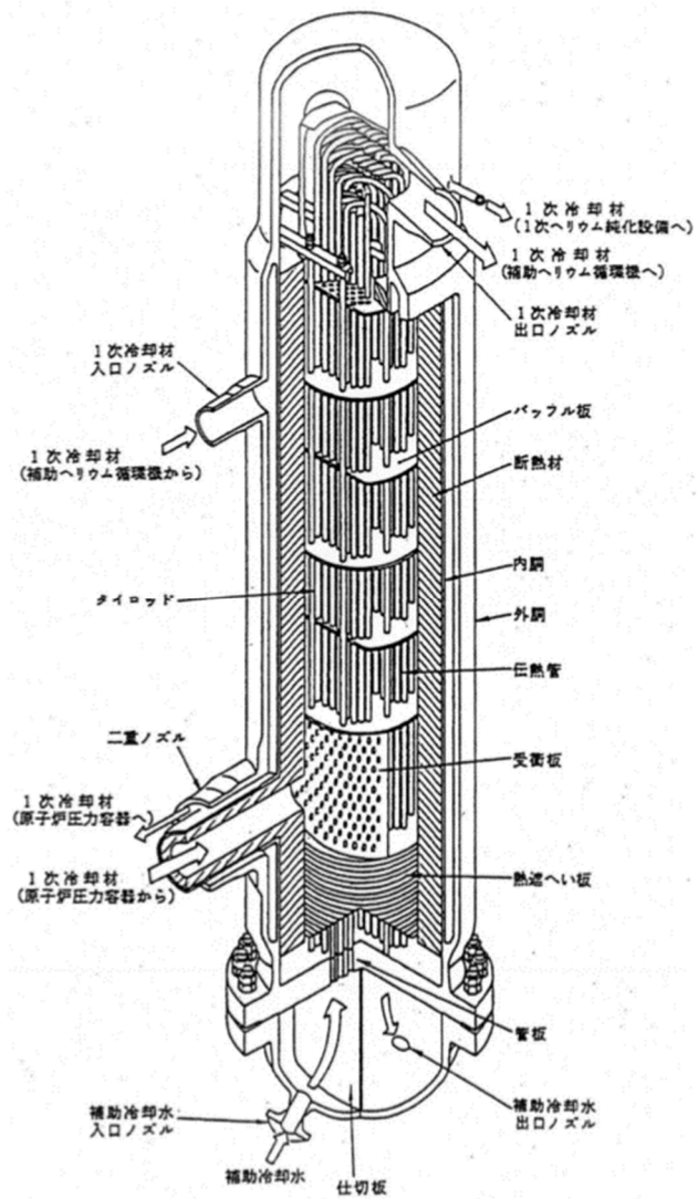
図2 補助冷却器鳥瞰図 (HTR 設置許可申請書より)
