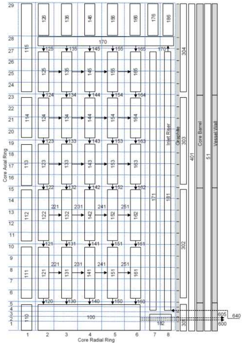
図 8 PBMR-400 の原子炉圧力容器（炉心部と圧力容器）の MELCOR 解析モデル
