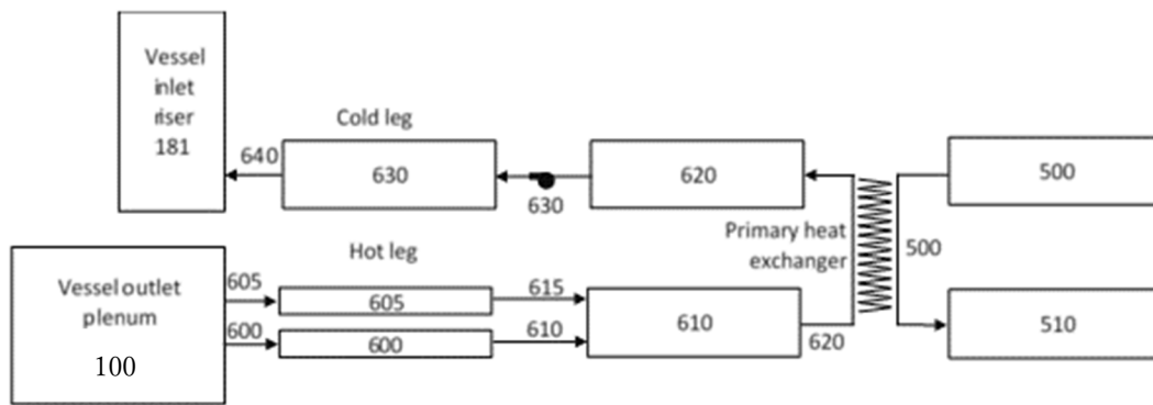
図 9 PBMR-400 の1次系、2次系解析モデル
