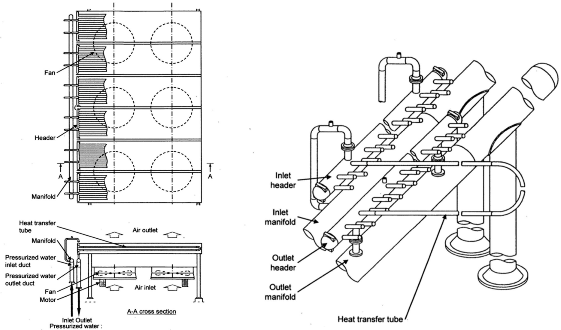
図4 主冷却系用空気冷却器の構造図 (JAERI-Tech 2005-041 より)
