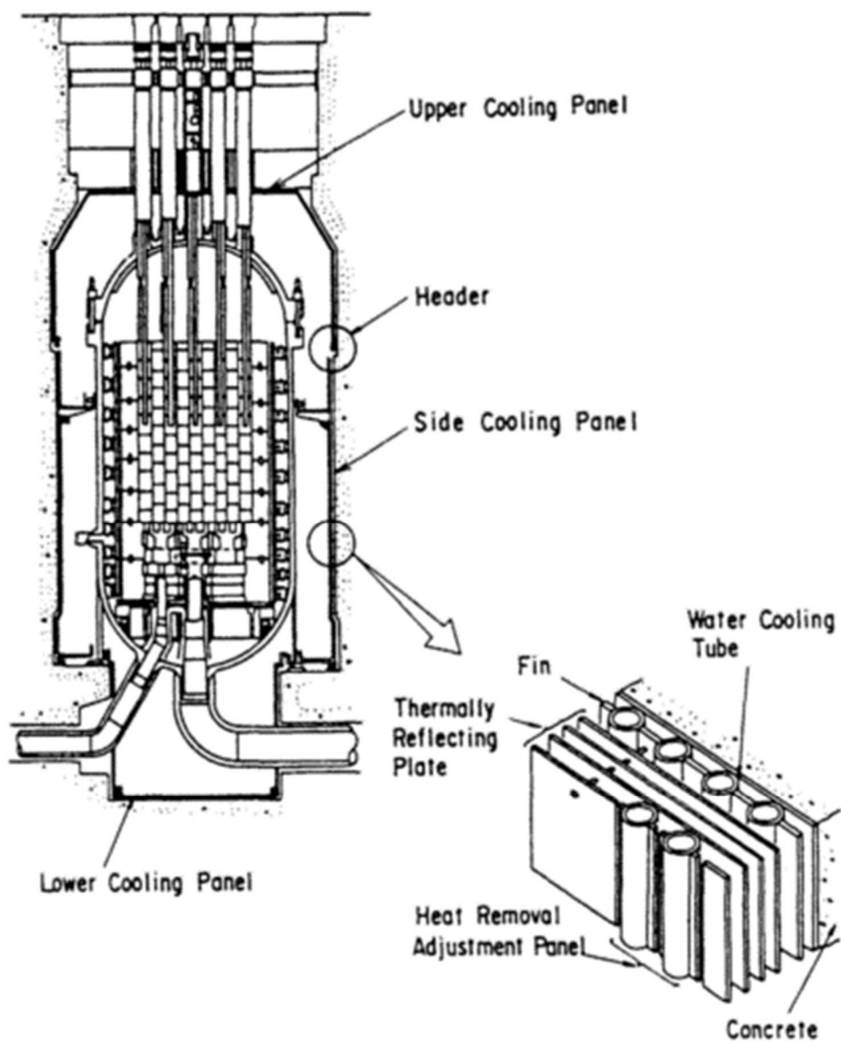
図 11 炉容器壁冷却系の概念
