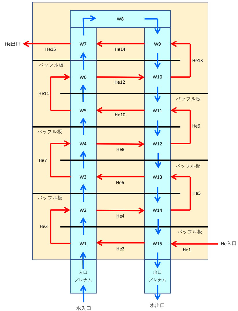
図3 補助冷却器の解析モデル概念
