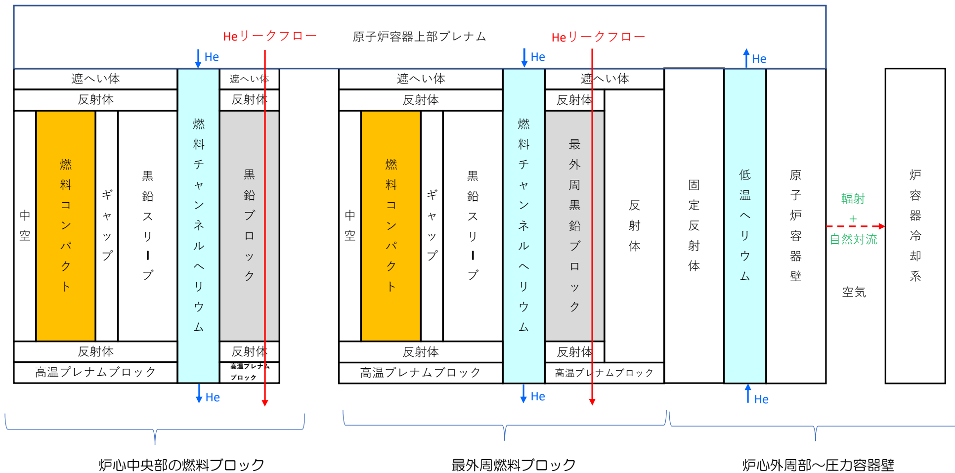
図6 原子炉解析モデルの改良
