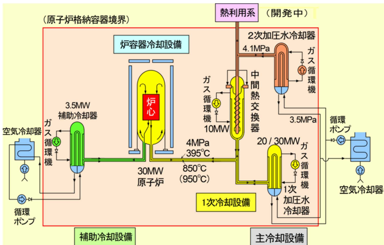
図1 HTTRの原子炉冷却系概念 (第35回核燃料施設等の新規制基準適合性に係る審査会合 資料1より)
