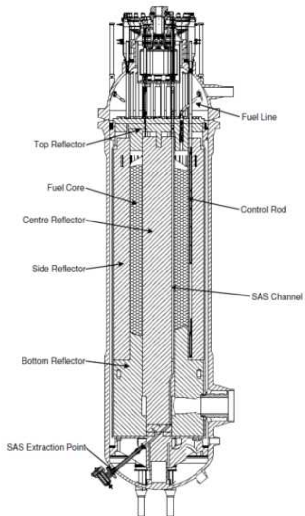
図7 PBMR-400 の原子炉圧力容器の構造 (SANDIA REPORT(SAND2022-2750 Rev.1)より)
