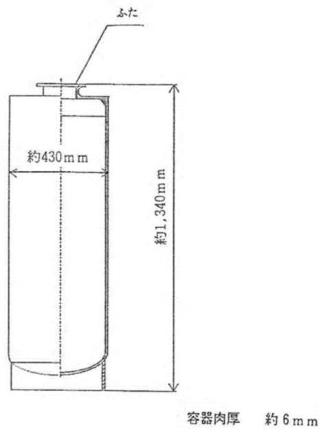
図2 ガラス固化体外観形状 (出典：再処理事業変更許可申請書添付書類六)
