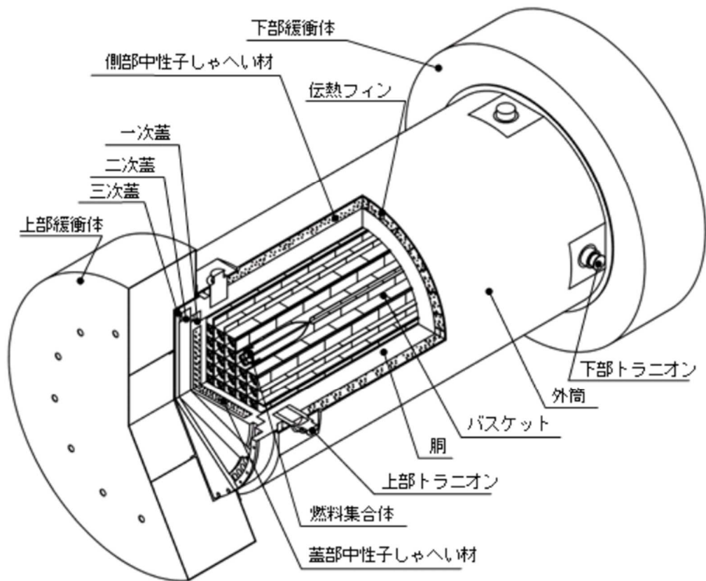
図1 金属キャスクの上部一部カットの方法と内部の可視化のイメージ (出典：「使用済燃料中間貯蔵に係る貯蔵後輸送の安全性確保方策について」、 平成22年2月3日、輸送物技術顧問会、
