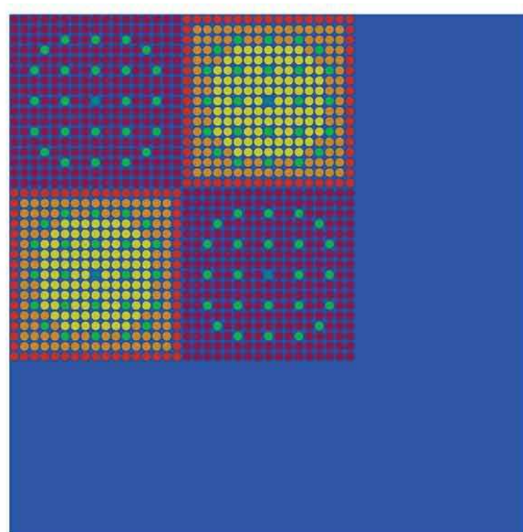
図3 反射体付き燃料集合体体系
