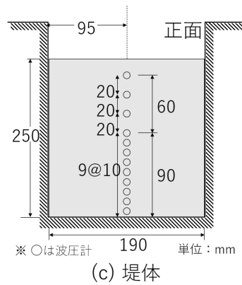
図1 水路及び堤体の概要
