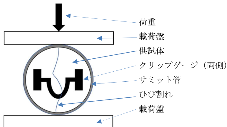
図1 ひび割れ導入の試験機
