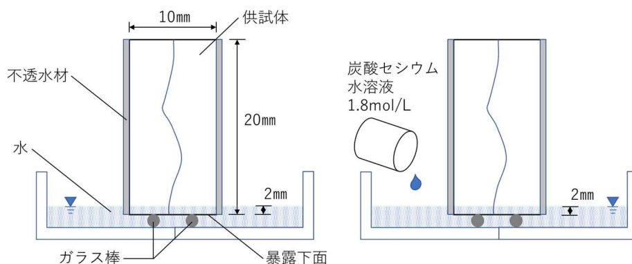
図2 トレーサー浸透の概念
