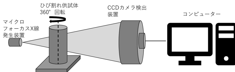
図3 X線CTによるひび割れ幅計測のイメージ
