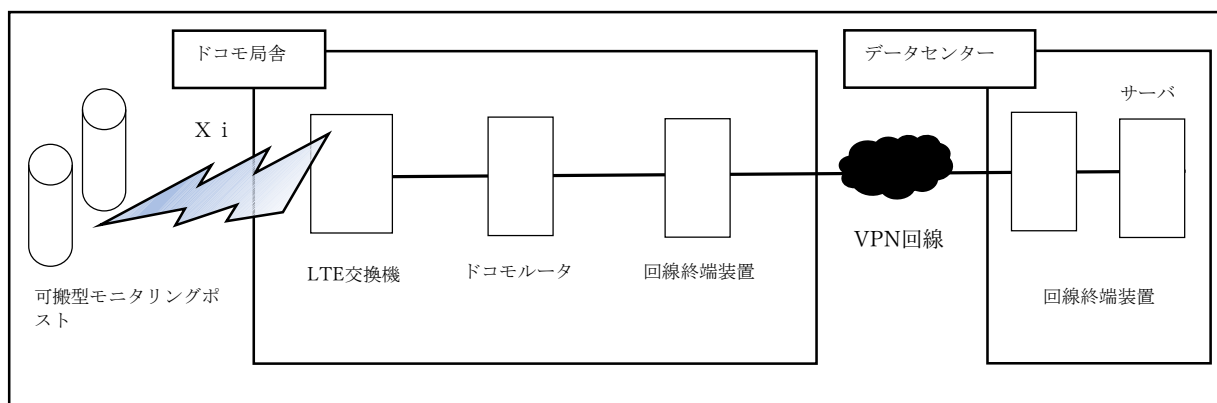
概略構成図
