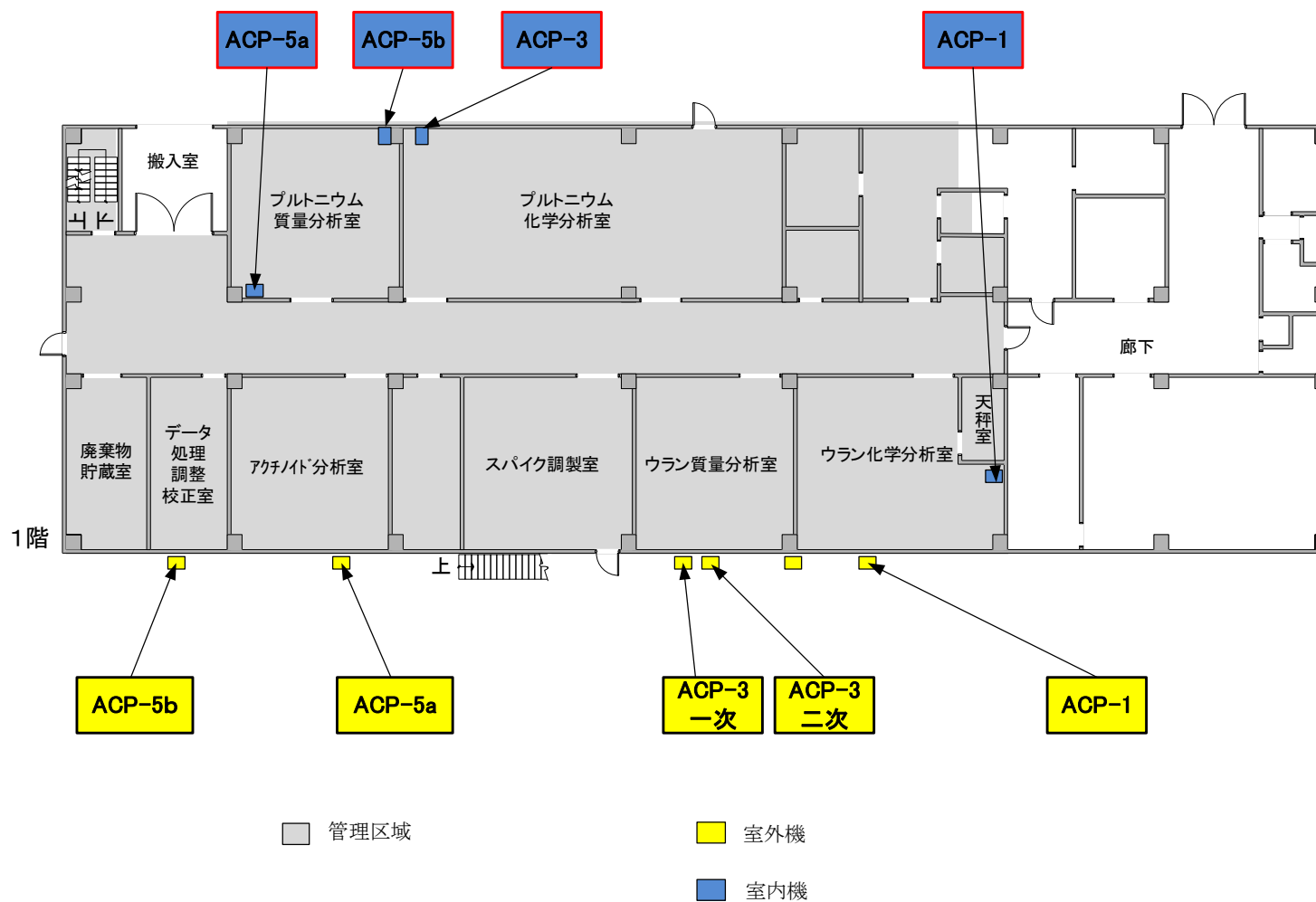
新分析棟空調設備の更新工事 空調設備配置図
