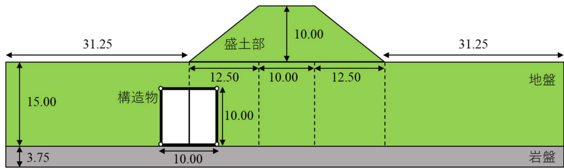
図 1※ モデルのイメージ（基本解析モデル 1）
