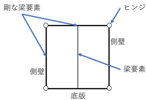
図 3※ モデルのイメージ（構造物）
