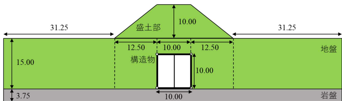
図 2※ モデルのイメージ（基本解析モデル 2）
