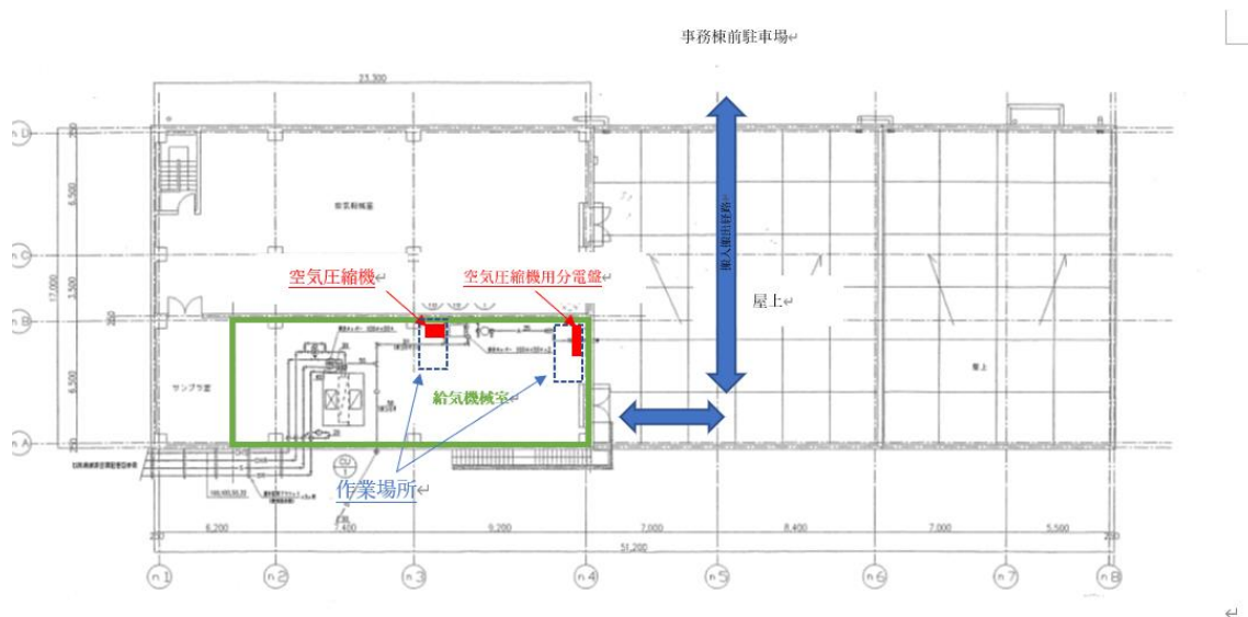
新分析棟 2 階 空気圧縮機 配置図
