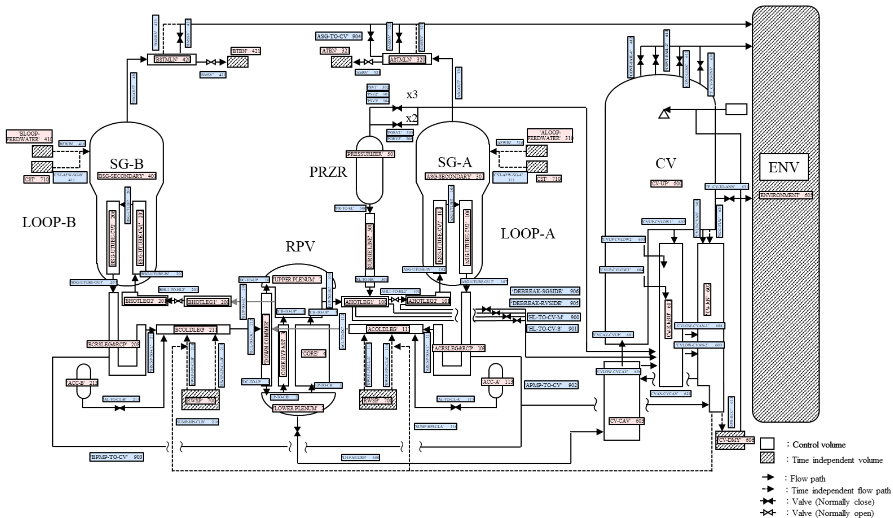
図 4.1 代表 PWR モデルのノード分割例 (Control volume : 約 70, Flow path : 約 100, HS : 約 130)
