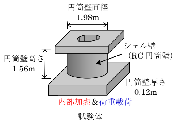
図2 RC円筒壁試験体のイメージ
