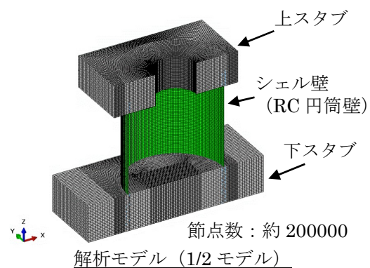
図3 RC円筒壁の解析モデル
