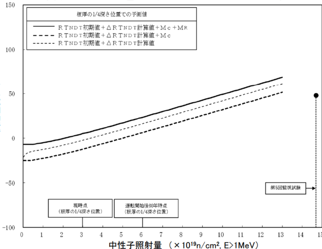
高浜3号炉 第5回監視試験で得られた 関連温度実測値(母材)に対する分析結果
