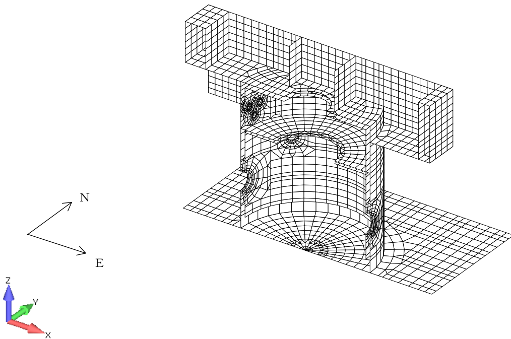
(b) 全体断面図 (EW 方向断面)
