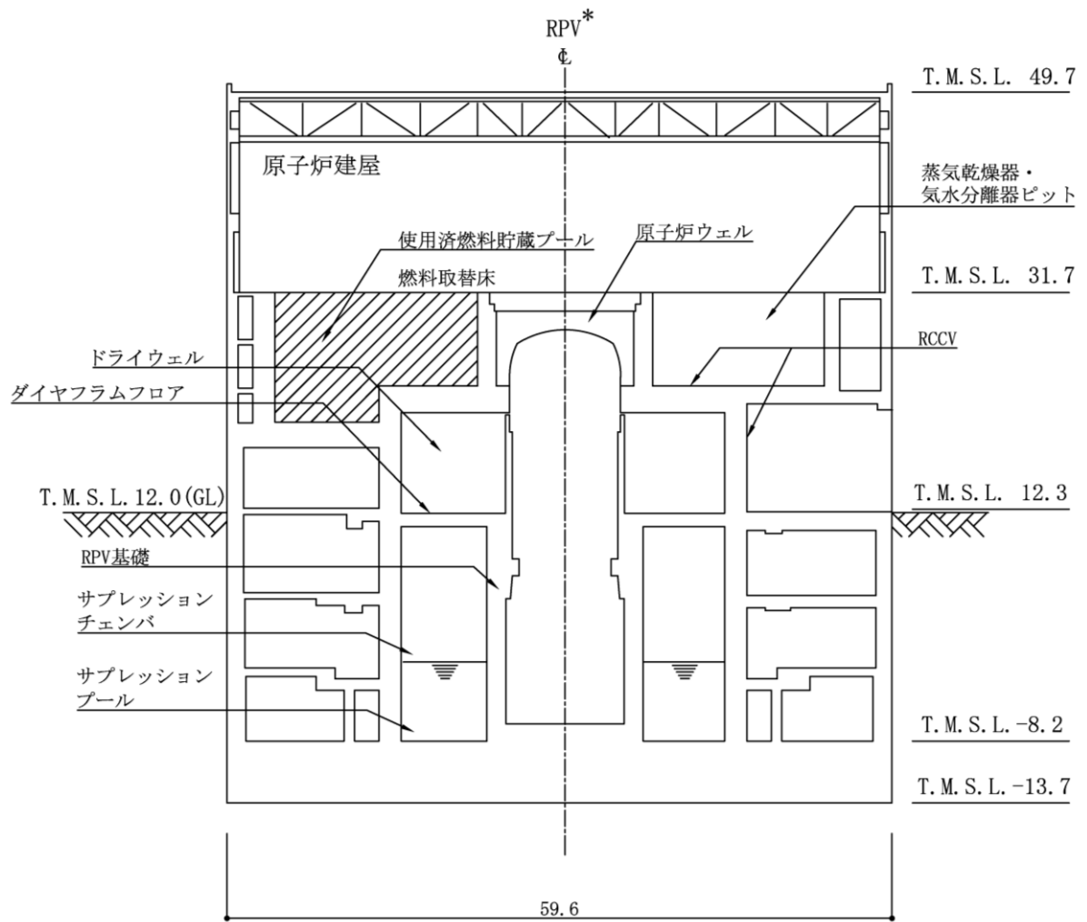
図 2-3 使用済燃料貯蔵プール及びキャスクピットを含む原子炉建屋の概略断面図 (A-A 断面) (単位：m)
