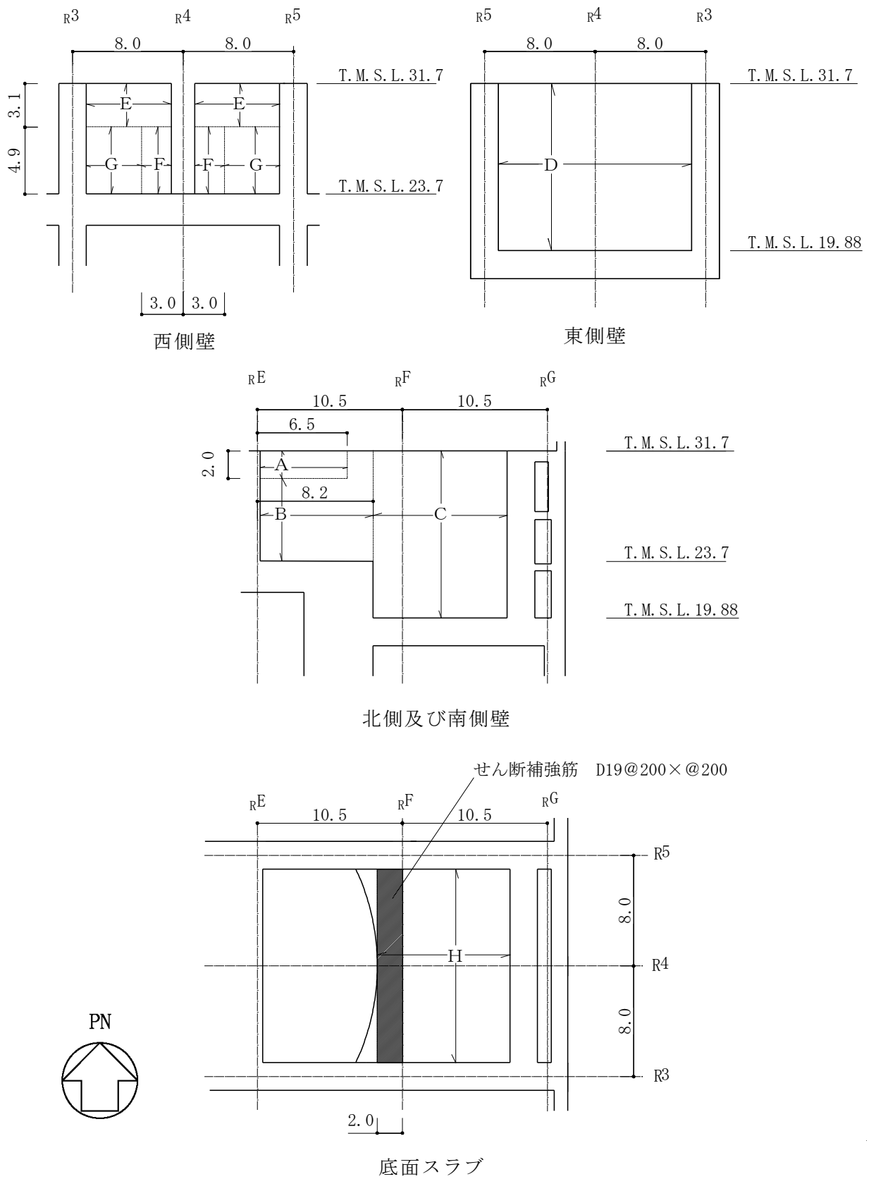
図 4-1 配筋領域図 (単位 : m)
