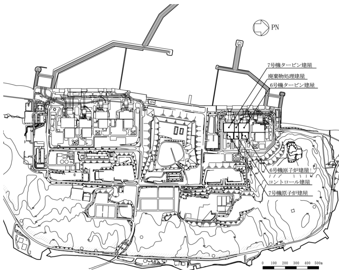
図 2-1 使用済燃料貯蔵プール及びキャスクピットを含む原子炉建屋の設置位置
