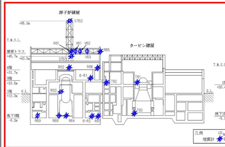
(2) 断面図
