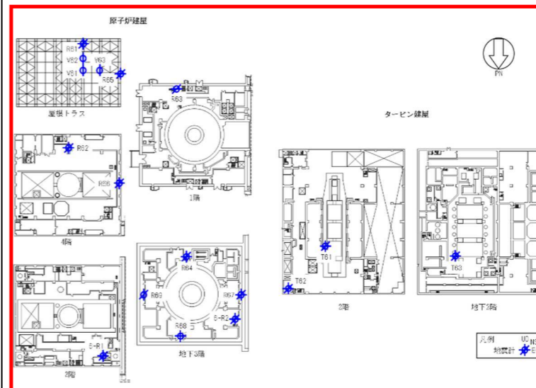
(1) 平面図
