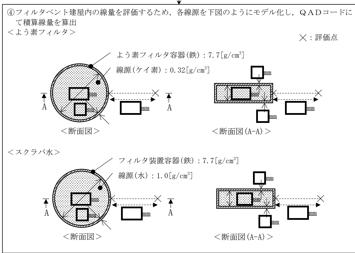
図1 フィルタベント遮蔽壁の遮蔽体表面における入射線量の評価のフロー図 (1/3)
