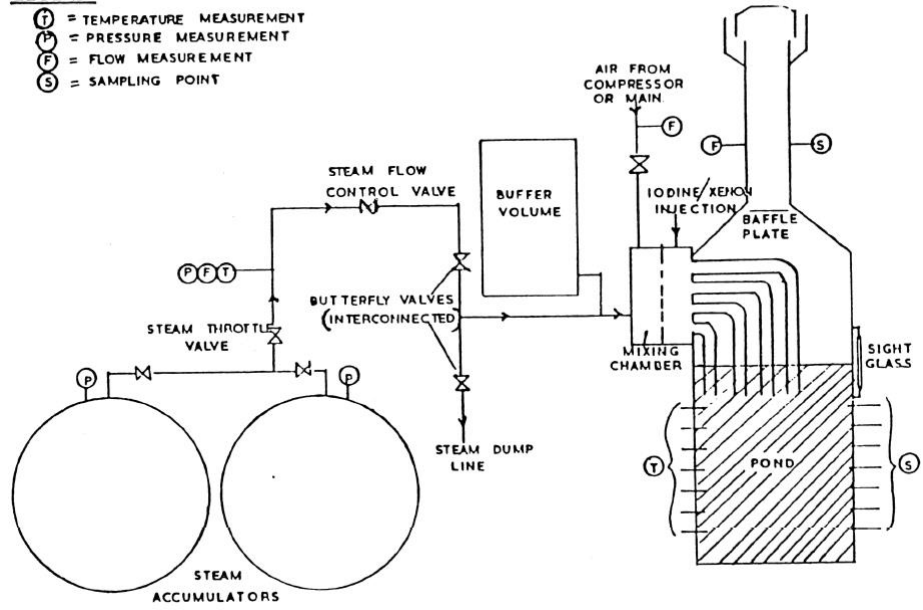
図2 UKAEA 実験体系
