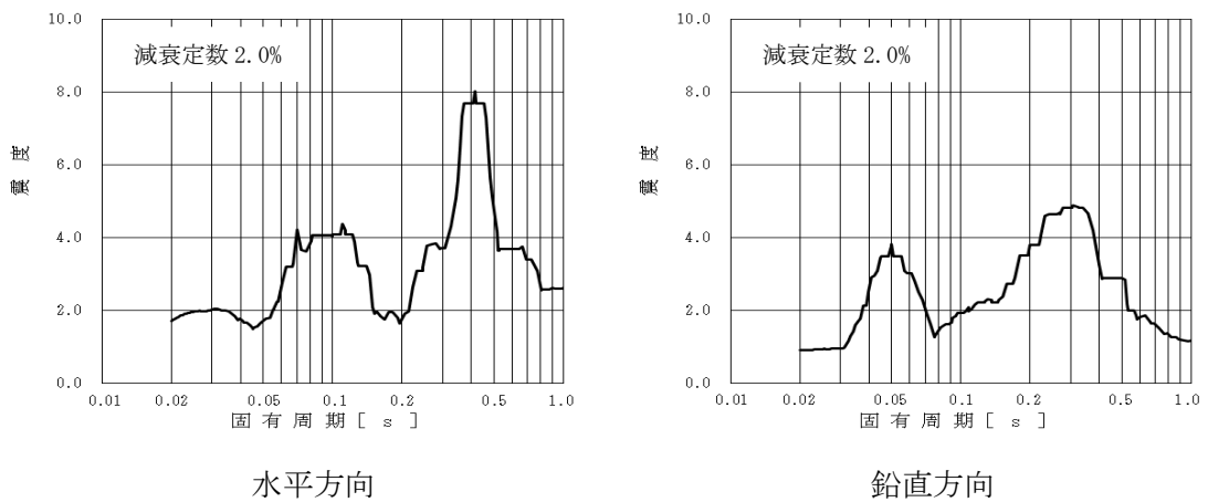
図 3(1) 原子炉遮蔽壁 (T. M. S. L. 18.100m) の検討用床応答曲線 (減衰定数 2.0%) (床応答スペクトルの計算範囲を 50Hz として作成)
