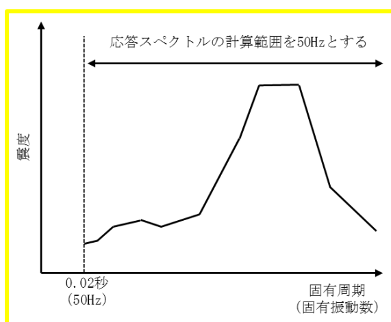
図 1(1) 計算範囲を 50Hz までとした床応答曲線 (イメージ図)
