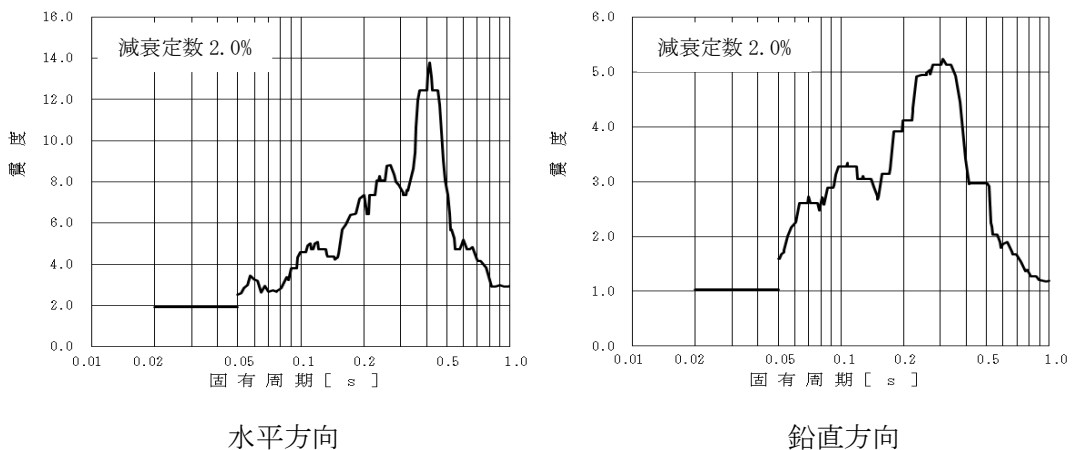
図 3(2) 原子炉建屋 (T. M. S. L. 49.700m) の設計用床応答曲線 (減衰定数 2.0%) (床応答スペクトルの計算を 20Hz とし、20Hz を超えた範囲は最大加速度として作成)
