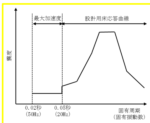
図 1(2) 20Hz 以降を最大加速度とした床応答曲線 (イメージ図)
