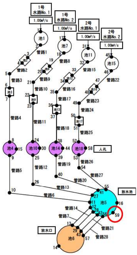
損傷 I (沈下) を考慮した管路解析モデル図 (健全地形と同じモデル)
