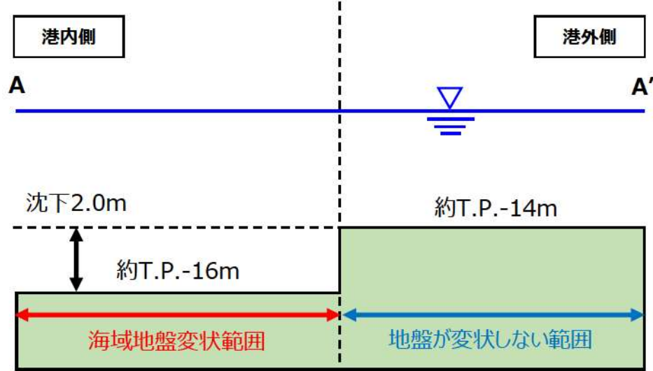
A-A'断面図
