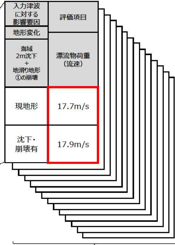
波源K 健全地形モデル以外のケース (19ケース)
