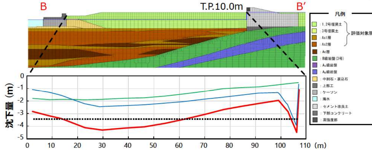
緑線 : 揺すり込み及び過剰間隙水圧消散に伴う沈下量【①】 青線 : 基準地震動による液状化に伴う側方流動による沈下量【②】 赤線 : 津波評価における沈下量【①+②】 (..... : 平均沈下量 = 3.32m)
