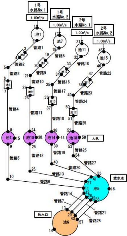
健全地形の管路解析モデル図
