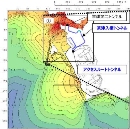
最大水位上昇量分布図※1
