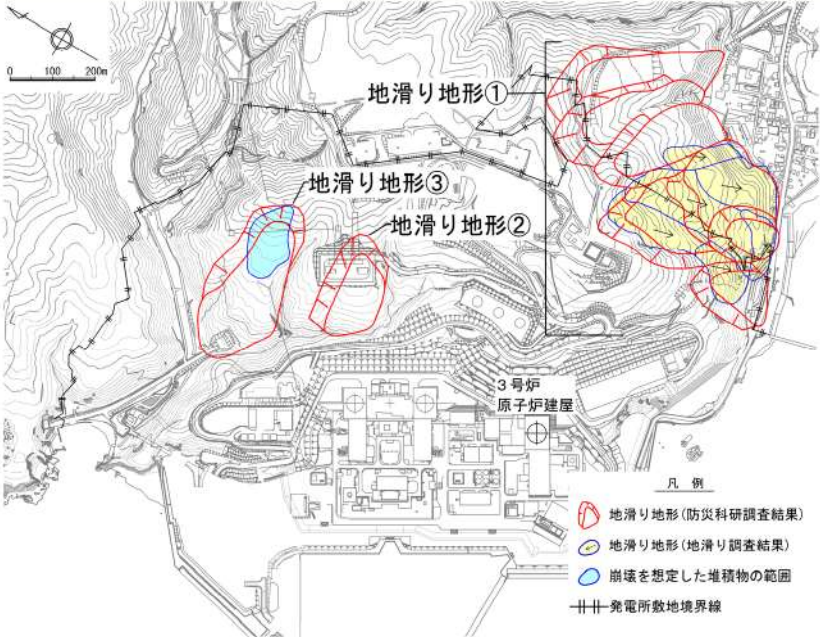
発電所背後の斜面に見られる地滑り地形位置図 「第6条：外部からの衝撃による損傷の防止(外部事象の考慮について)」(一部修正)
