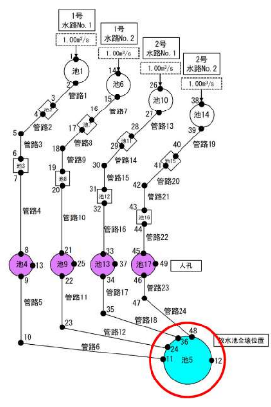
損傷 IV (部材損傷(放水池全壊)) を考慮した管路解析モデル図
