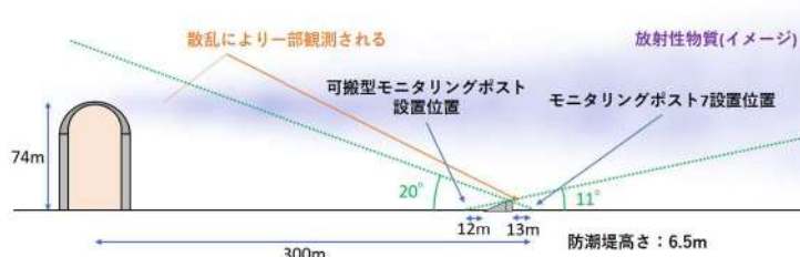
第7図 クラウドシャイン線の観測への影響確認（防潮堤高さ 6.5m）
