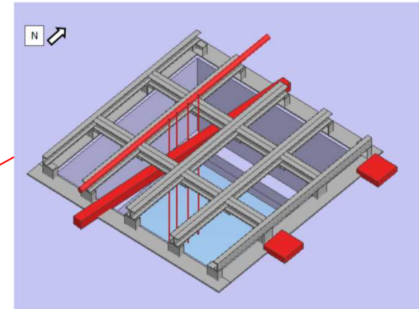
開口部①閉止イメージ（基礎部）
