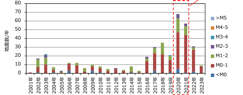
地震発生回数の年別時間変化(2001年~2023年※, 深さ40km以浅) ※2001年は10月1日~12月31日, 2023年は1月1日~3月31日のデータを掲載。
