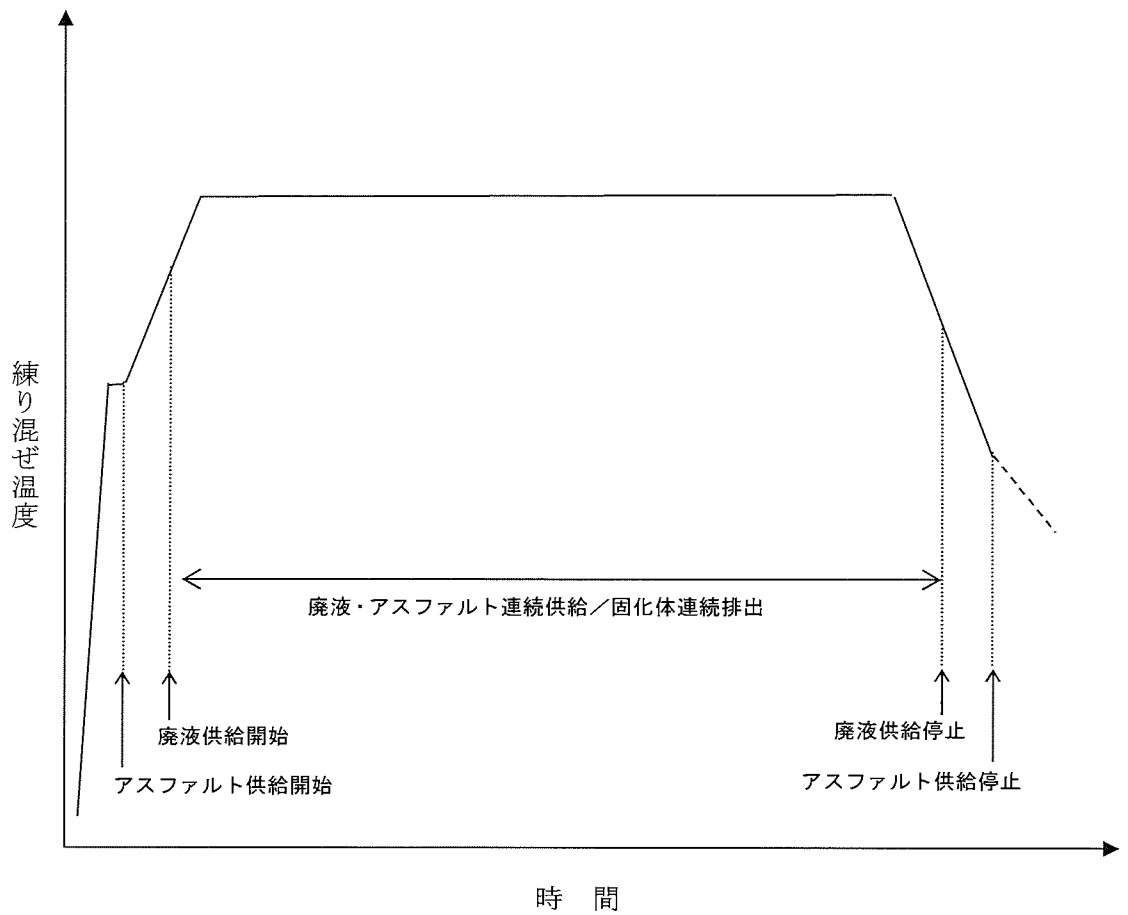
図-2 アスファルト固化装置運転工程
