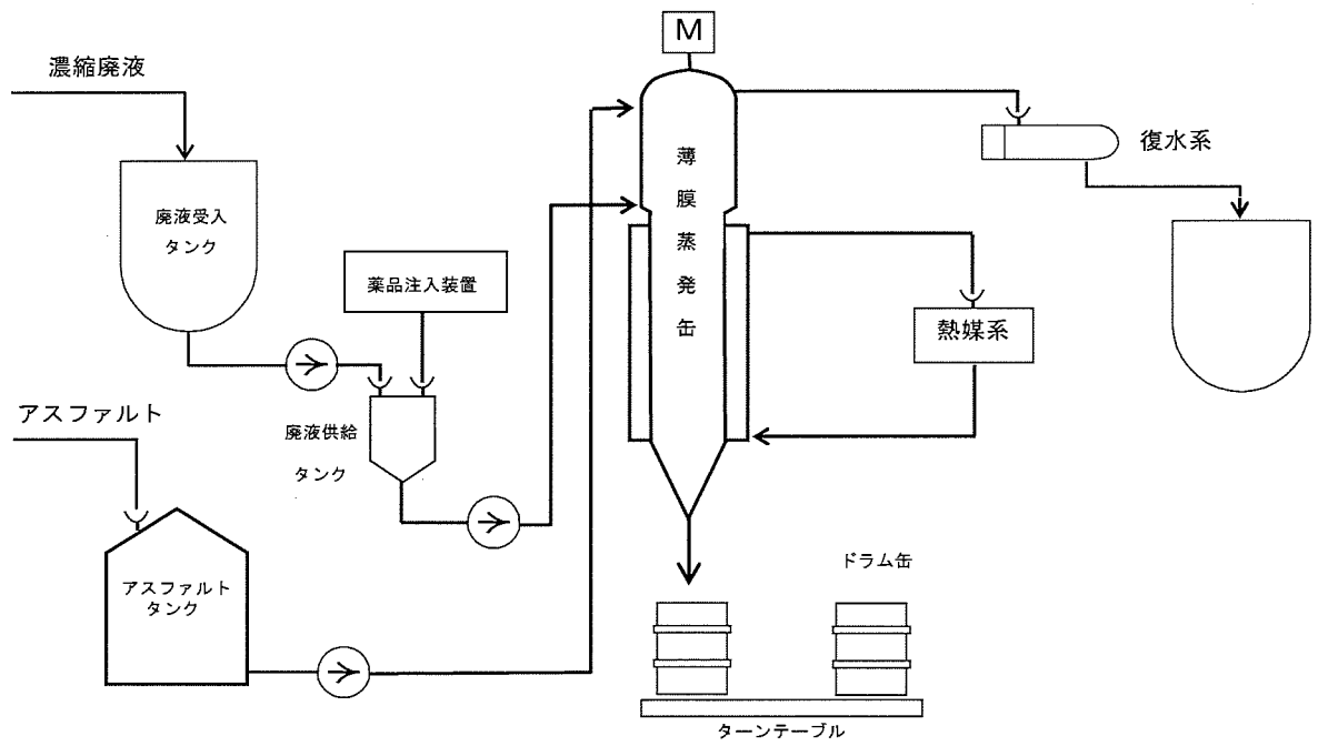
図-1 アスファルト固化処理装置概念図
