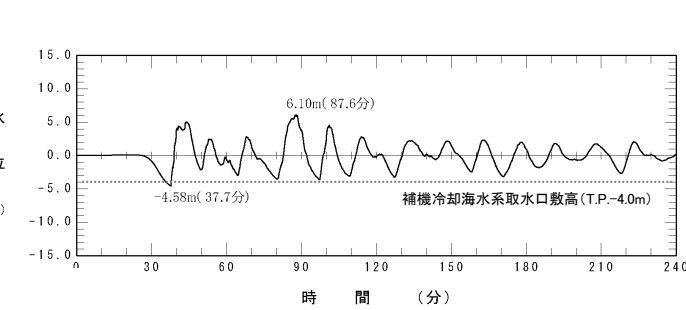
補機冷却海水系取水口前面における 水位時刻歴波形※1, 2
