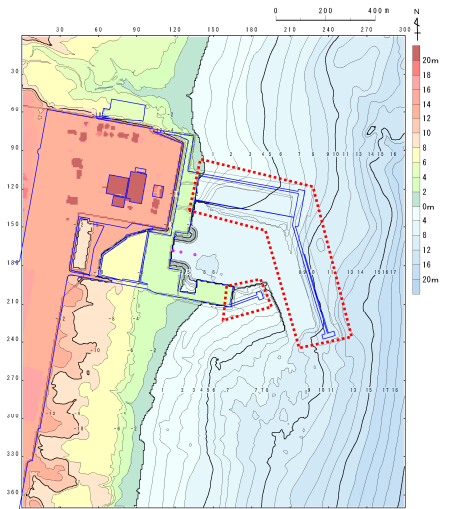
防波堤無し
