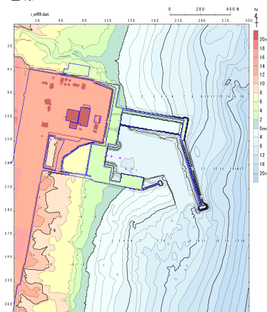
防波堤有り
