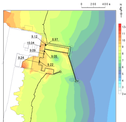
津波地震
