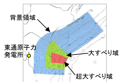
特性化モデル②
