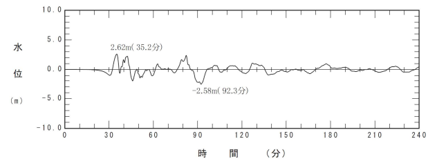
津波地震
