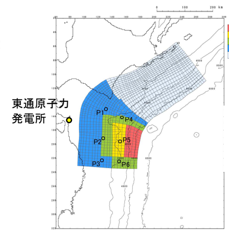
基準断層モデル③
