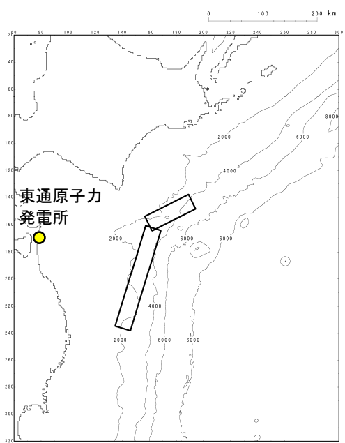
波源位置
