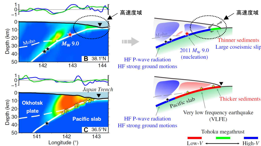
プレート境界におけるP波速度分布とそのイメージ (Liu and Zhao(2018)に一部加筆)
