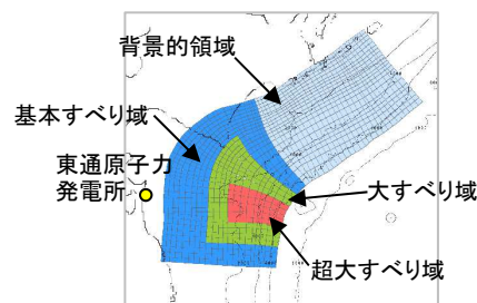
特性化モデル③
