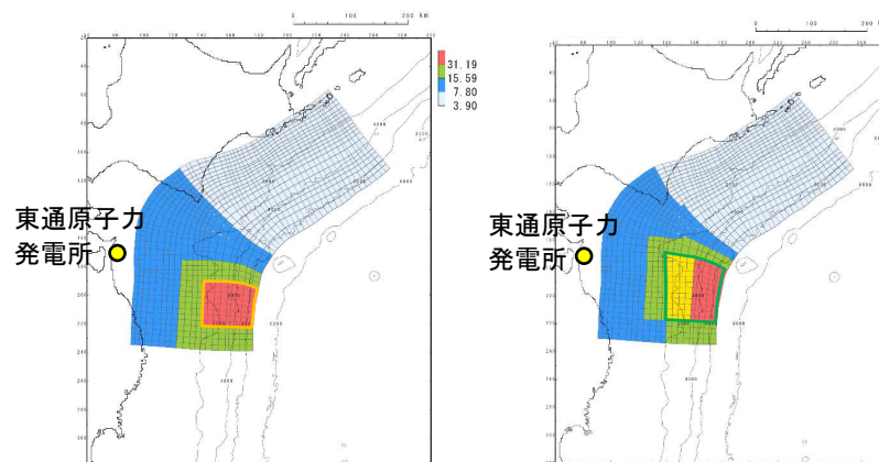
特性化モデル③ (南へ約100km移動)
