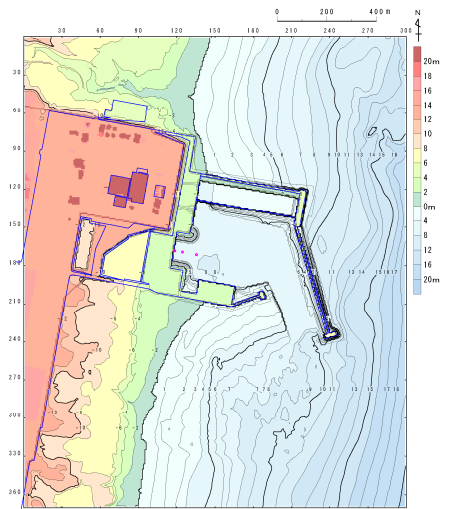
防波堤有り
