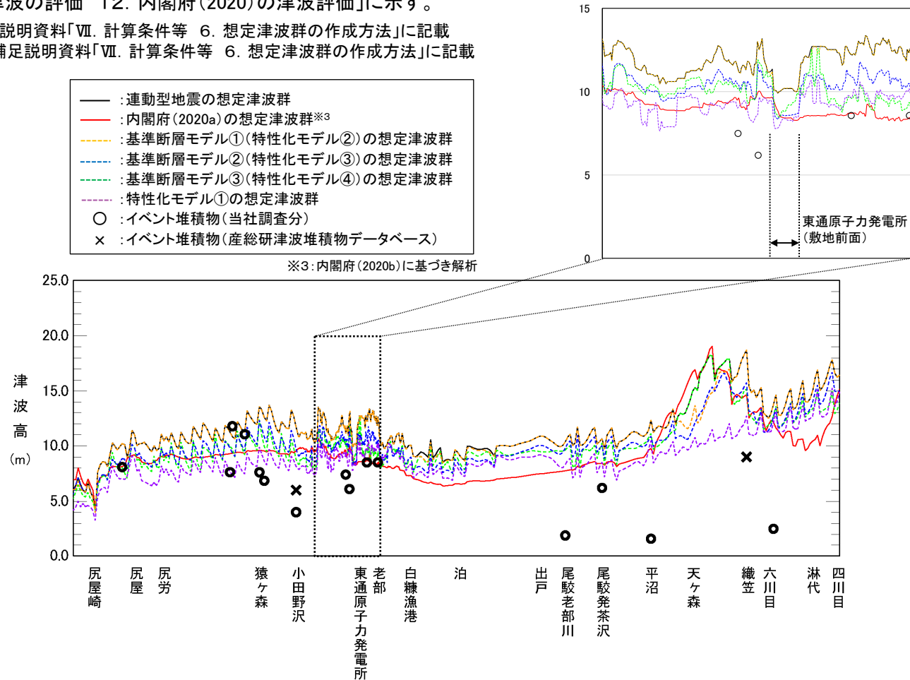
青森県北部太平洋沿岸の汀線位置における十勝沖・根室沖から岩手県沖北部の連動型地震の想定津波群とイベント堆積物及び内閣府(2020a)による日本海溝(三陸・日高沖)モデルの想定津波群の比較 ※4
