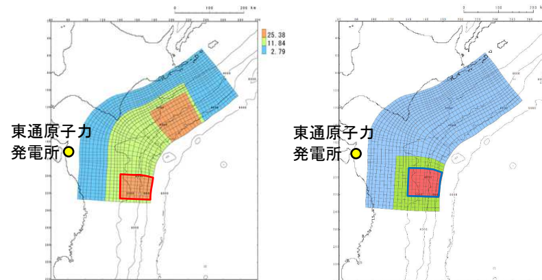
特性化モデル① (南へ約50km移動)
