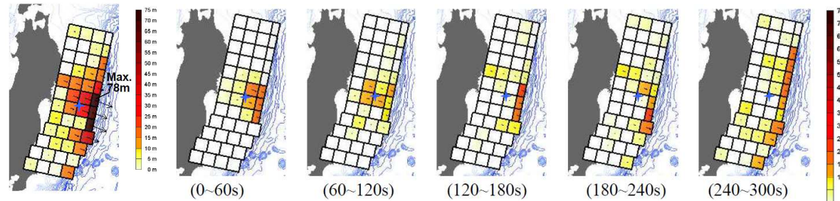
すべり量分布(合計) (確定波源モデル)
