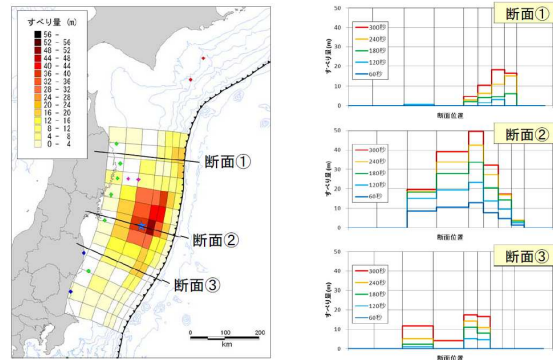
すべり量分布(合計)
