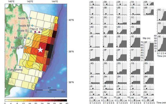
すべり量分布(合計)
