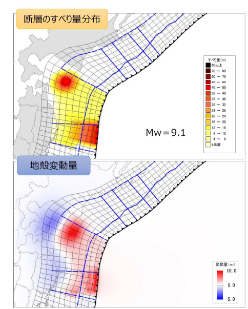
内閣府の津波波源モデル 日本海溝(三陸・日高沖)モデル(Mw9.1) (内閣府(2020a))
