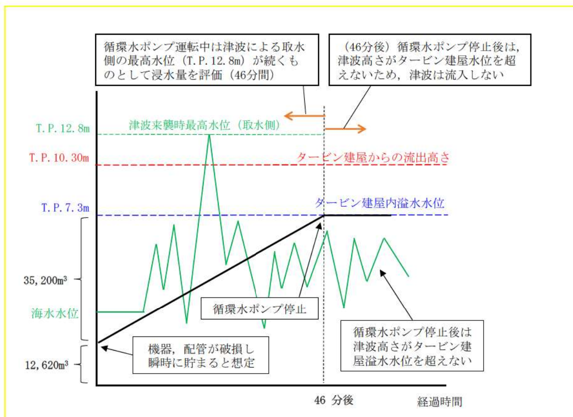
図 4 タービン建屋内の溢水水位イメージ
