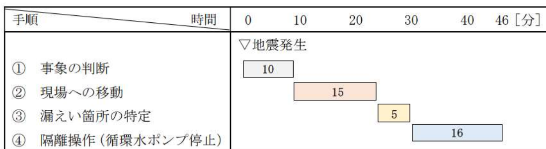
図2 循環水ポンプ停止までの時間
