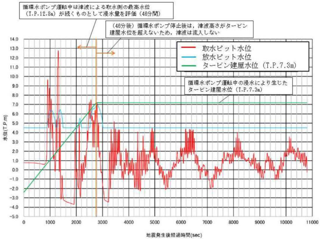
図6 取水側及び放水ピットの水位波形
