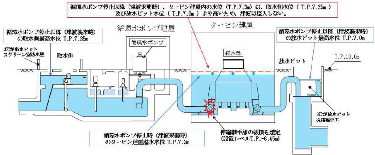
図7 循環水ポンプ停止以降（津波来襲時）のタービン建屋内水位と取水側水位及び放水ピット水位の概略図
