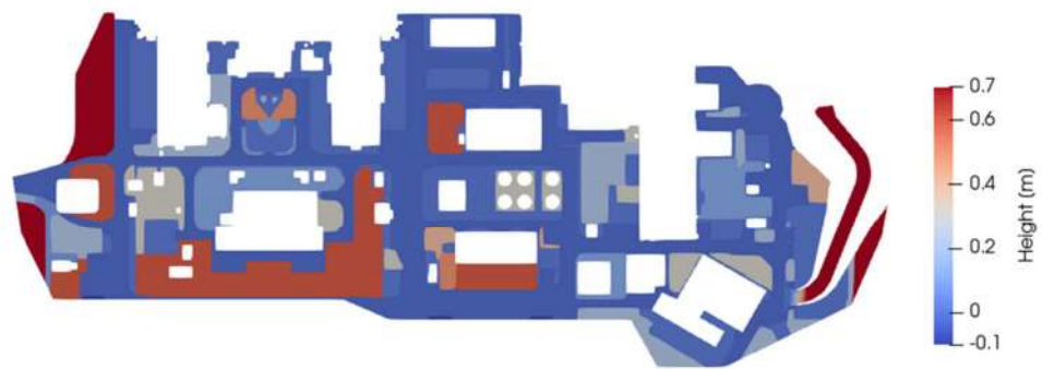
図2 敷地モデル
