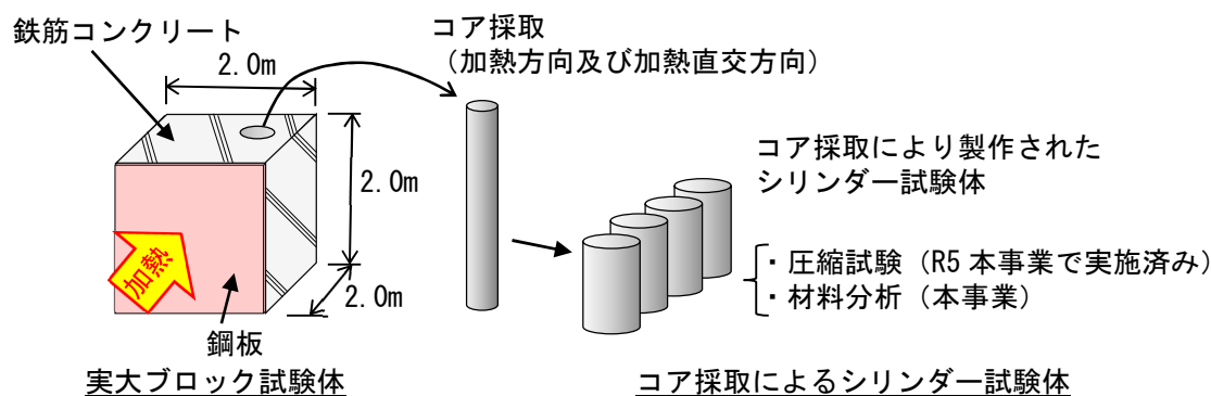
図2 実大ブロック試験体の分析イメージ
