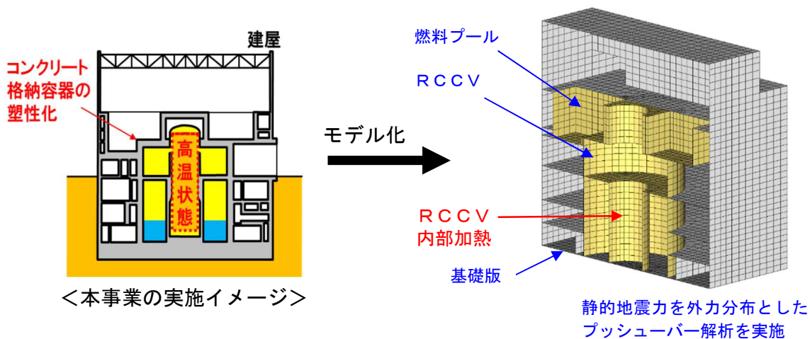
図5 仮想実機建屋モデルのイメージ
