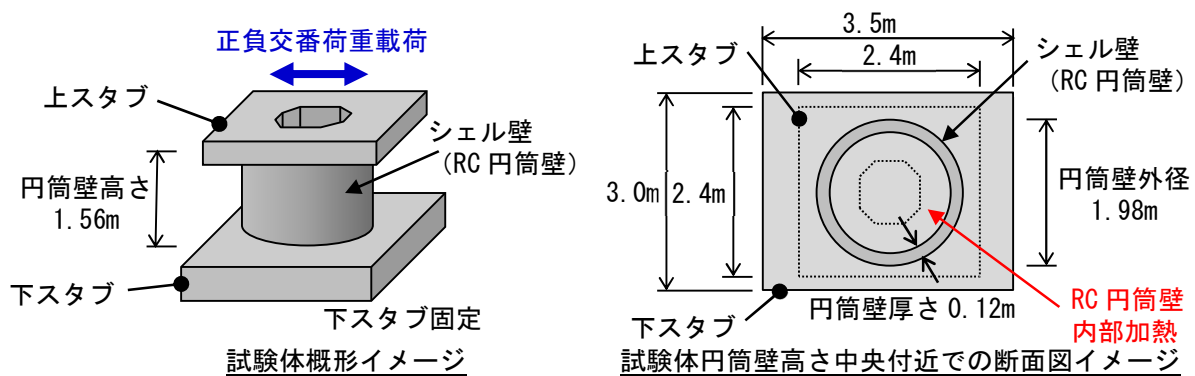
図3 RC円筒壁試験体のイメージ
