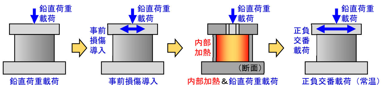
図4 RC円筒壁試験(事前損傷:有り)の試験フローのイメージ
