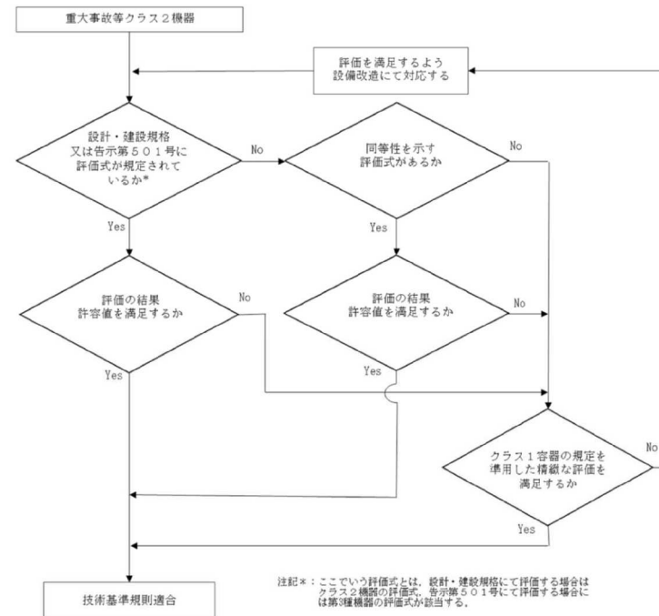
図 2-2 重大事故等クラス2機器の技術基準規則適合性確認フロー
