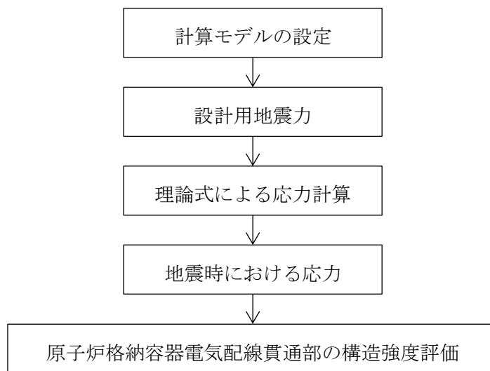
図2-1 原子炉格納容器電気配線貫通部の耐震評価フロー
