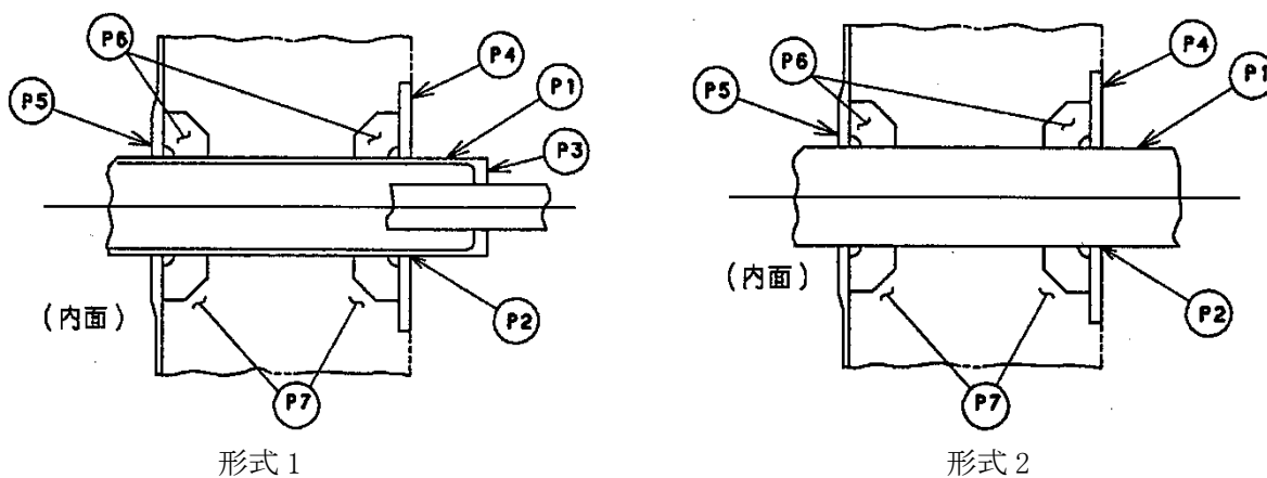
図 4-2 原子炉格納容器配管貫通部の応力評価点
