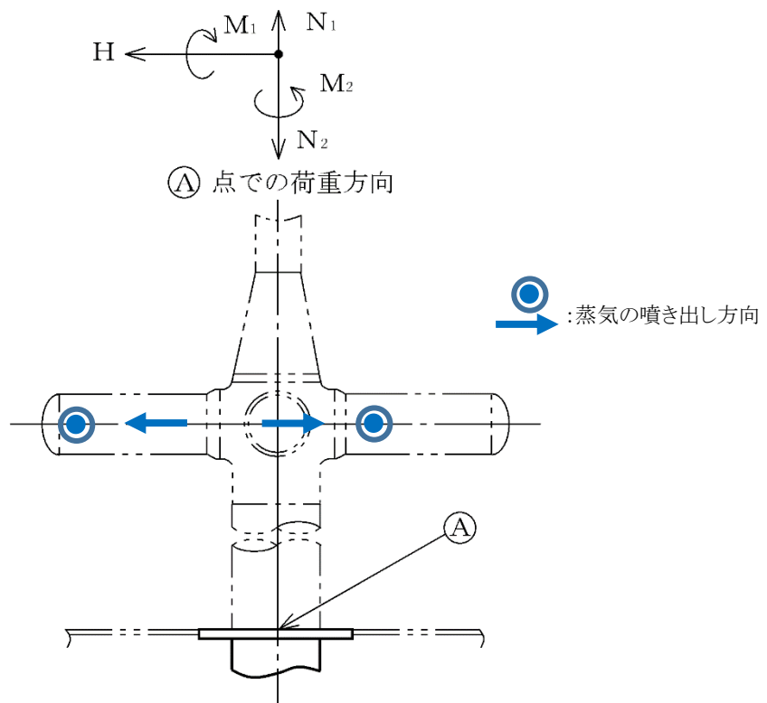
図 3-1 クエンチャサポート基礎における荷重方向
