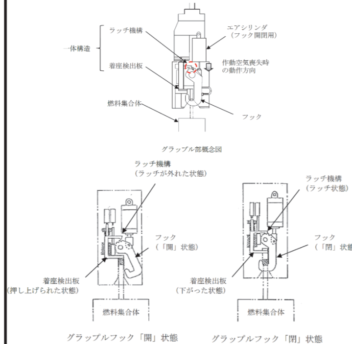
図3-1 グラップルの空気源喪失時にも燃料体等をつかむ構造
