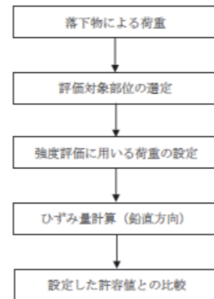
図5-4 燃料集合体の強度評価フロー
