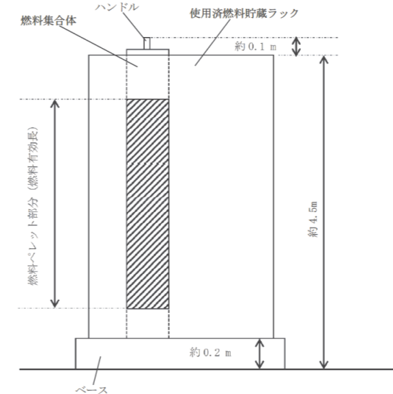
図5-3 燃料集合体及びラックの関係図
