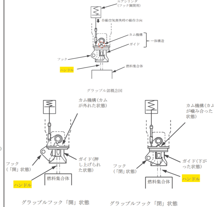
図3-1 グラップルの空気源喪失時にも燃料体等をつかむ構造
