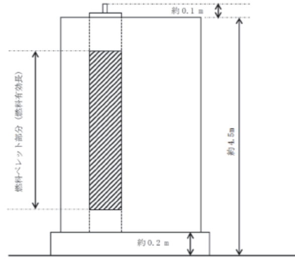
図5-3 燃料集合体及びラックの関係図
