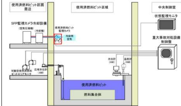
図1 使用済燃料ピット監視計器の概略図
