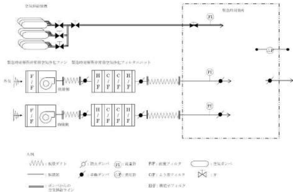
図5-2 緊急時対策所換気設備概要図
