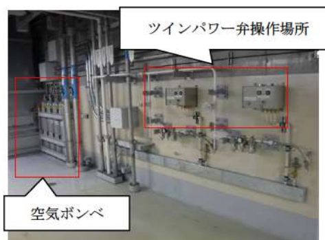
余熱除去ポンプ入口弁操作用可搬型空気ボンベ (原子炉補助建屋 T. P. 10. 3m)
